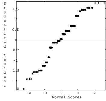
Fig. 1. Rankits plot
